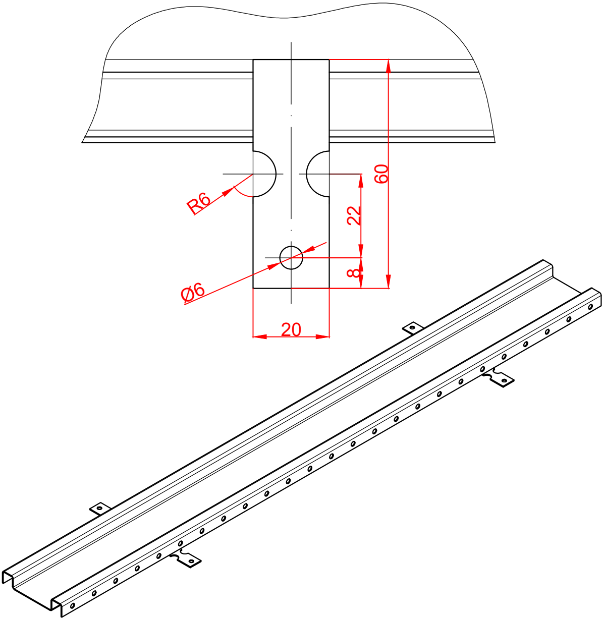
Б (1:1)
